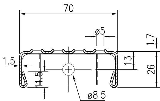
SCHNITT A-A
