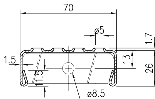
SCHNITT A-A
